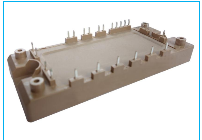
Rectifier+Brake+Inverter
