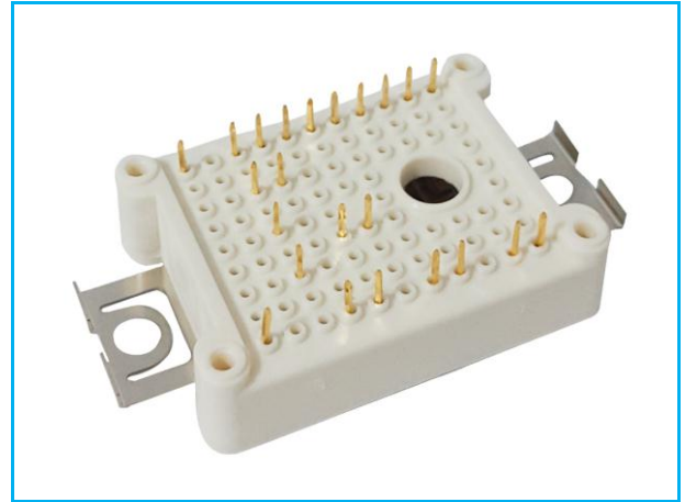
Rectifier+Brake+Inverter
